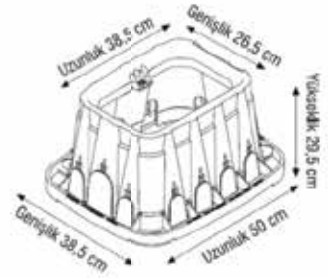
12 " VANA KUTUSU
