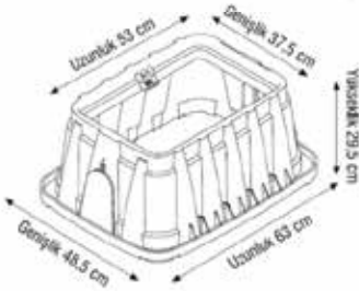
14 " VANA KUTUSU
