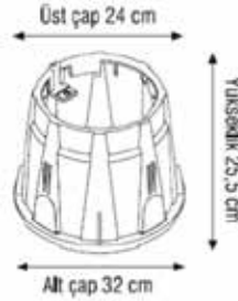
10 " VANA KUTUSU
