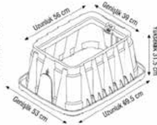
16 " VANA KUTUSU
